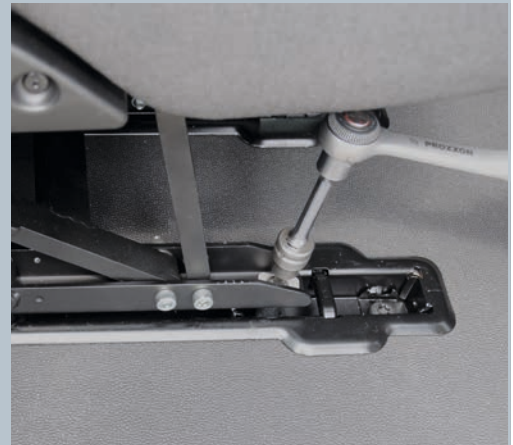
Die Sitzbefestigung erfolgt durch Einschrauben
